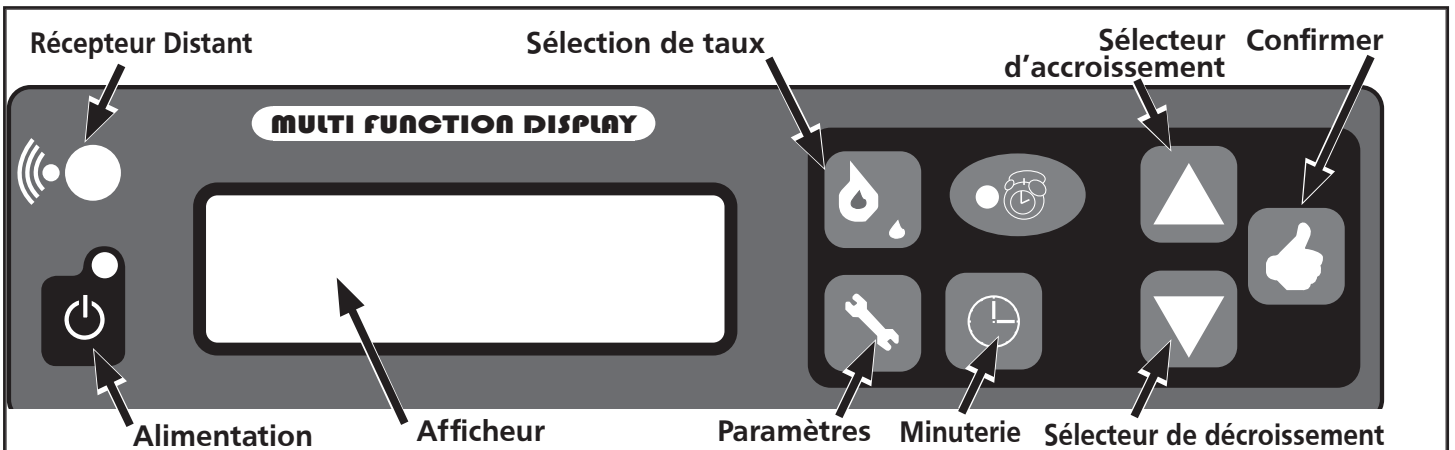
Figure 19a Panneau multi-fonction monté
