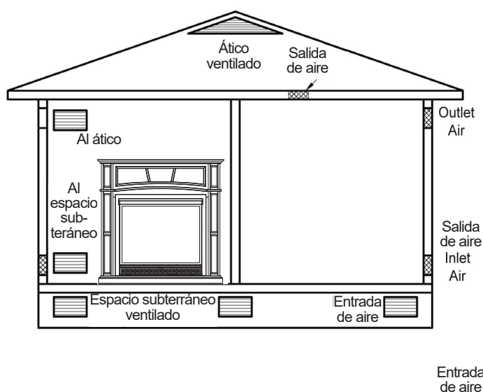
Fig. 5: aire de ventilación del exterior
