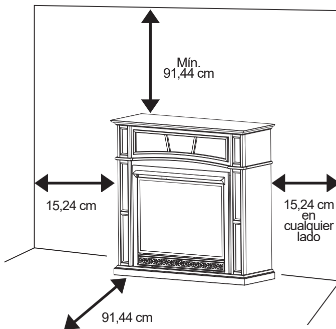
Fig. 6: distancia de separación mínima con materiales combustibles
