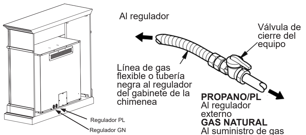
Fig. 11: conexión flexible de la línea de gas a la válvula de cierre del equipo
