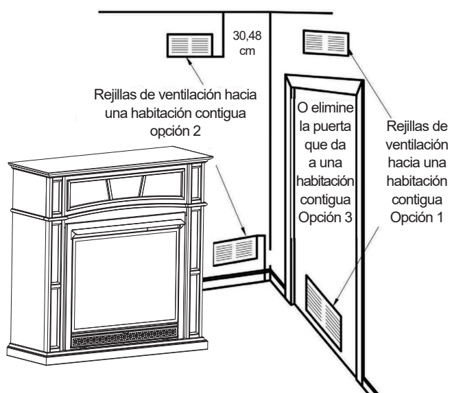
Fig. 4: aire de ventilación del interior del edificio
