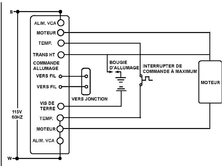
SCHÉMA DE CIRCUITS
