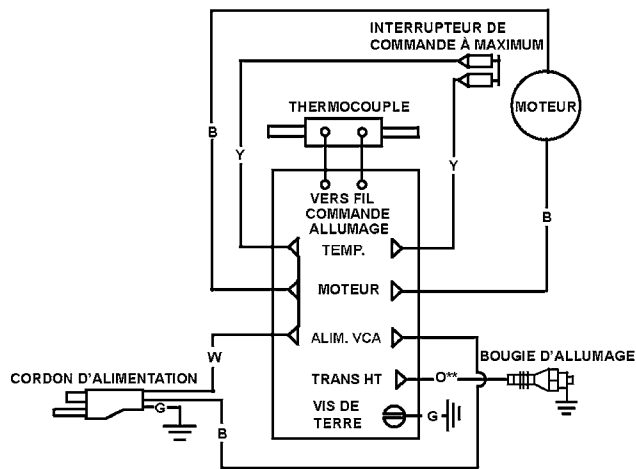
SCHEMA DE CONNEXION
