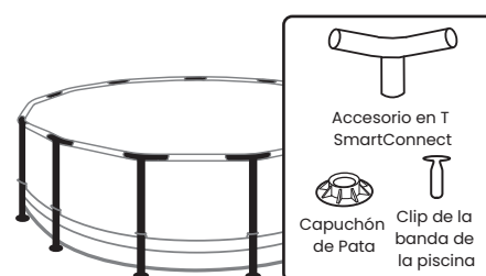
Piezas y accesorios en T SmartConnect
