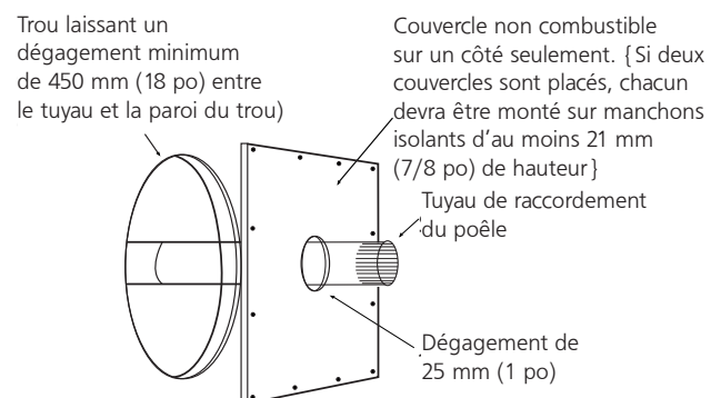
Figure 5 SEULEMENT UN TUYAU DE TRAVERSÉE CONFORME AUX NORMES CANADIENNES
