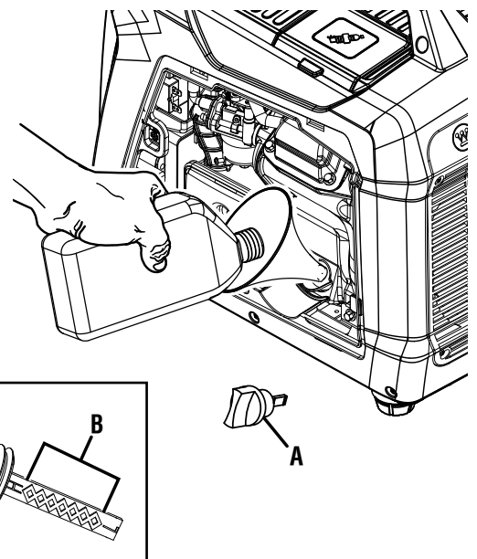
A - Jauge d'huile B - Plage de fonctionnement sécuritaire
