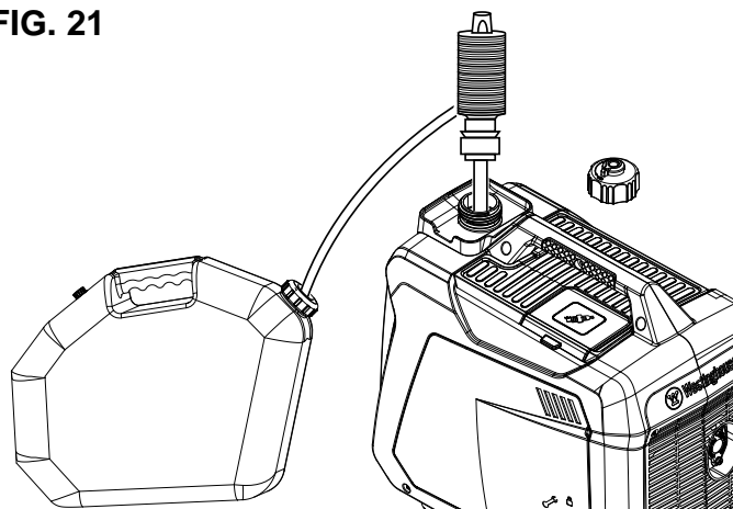
A - Apagado del motor/combustible
