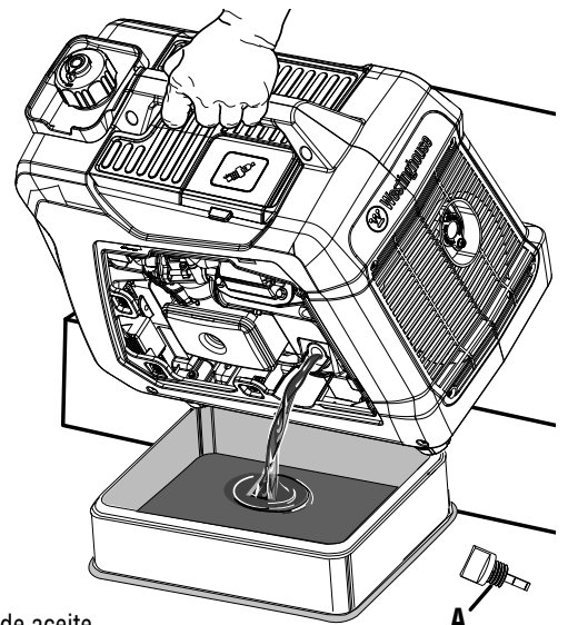
A - Varilla de nivel de aceite
