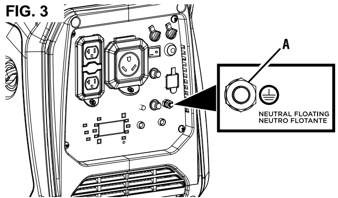
A - Borne mise à la terre
