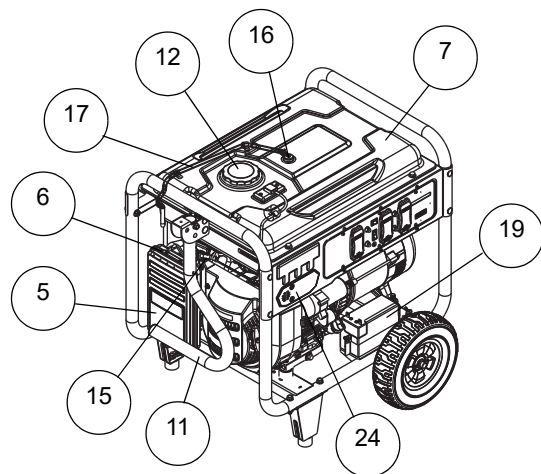
DXGNR 8000
