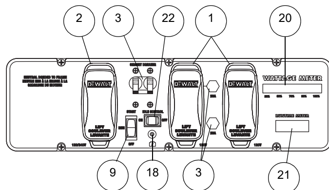
DXGNR 8000
