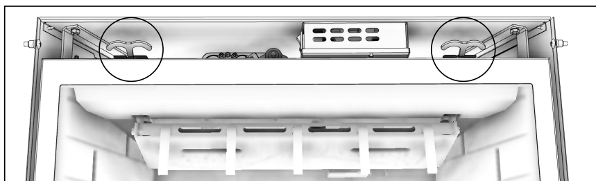
1. Localisez les deux (2) loquets à ressorts qui fixent l'assemblage vitré au bas de la boîte à combustion.
