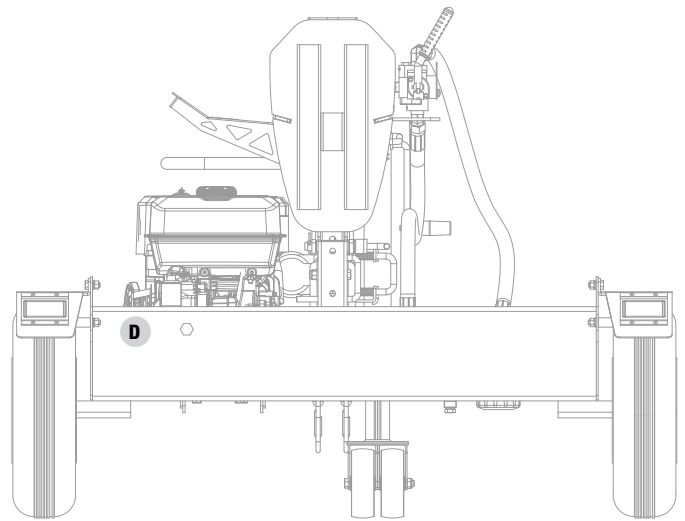
Vista trasera
