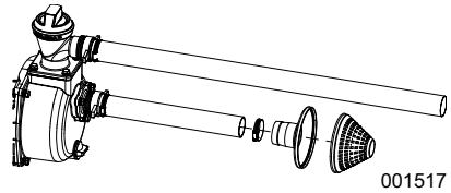
Figura 2-6. Conexión de filtro típica
