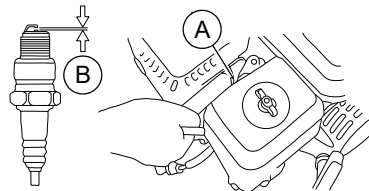
Figure 4-2. Entretien de la bougie d'allumage (image générique affichée)
