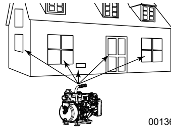
Figure 3-1. Dégagez un espace minimal de cinq pieds
