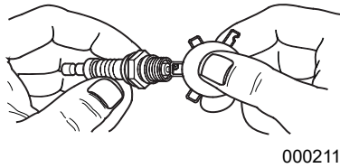
Figura 4-3. Separación de la bujía
