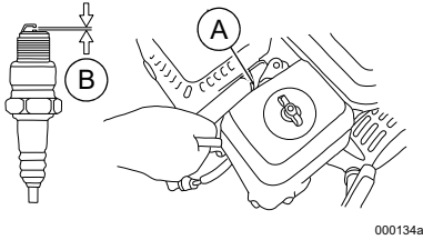
Figura 4-2. Mantenimiento de la bujía (se muestra imagen genérica)
