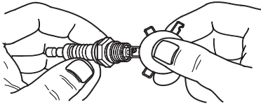
Figure 4-3. Écartement des électrodes de la bougie d'allumage
