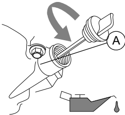
Figura 2-1. Sacar la varilla
