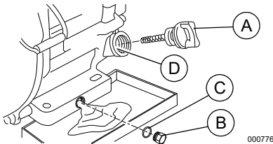
Figure 4-1. Vidange de l'huile moteur (image générique affichée)
