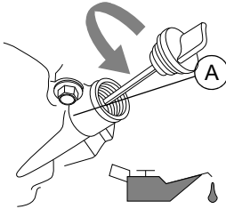
Figure 2-1. Retrait de la jauge
