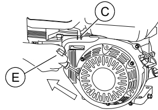
Figura 3-4. Arranque del motor con tirador y cuerda (se muestra imagen genérica)
