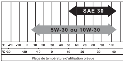
Figure 2-2. Huile recommandée
