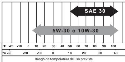
Figura 2-2. Aceite recomendado
