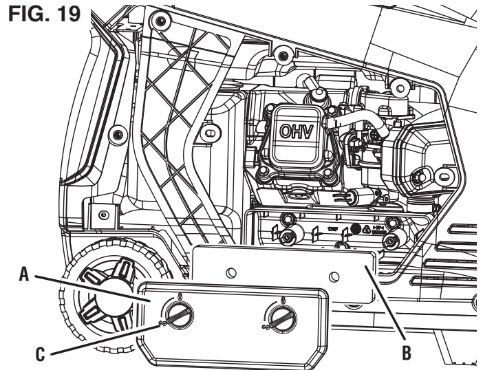
FIG. 19 A - Cubierta del filtro de aire B - Filtro de aire C - Perilla de bloqueo
