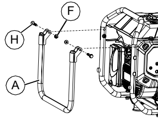
Figura 2-11. Asa de transporte
