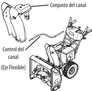
Control del Canal Superior (Eje Flexible) c/ Canal de Acero y Control de Inclinación de 2 Direcciones on página 42
