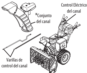
Control de Rotación del Canal Superior c/ Control Eléctrico de Rotación e Inclinación de 4 Direcciones on página 44
