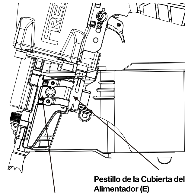
Cubierta del Alimentador (F)
