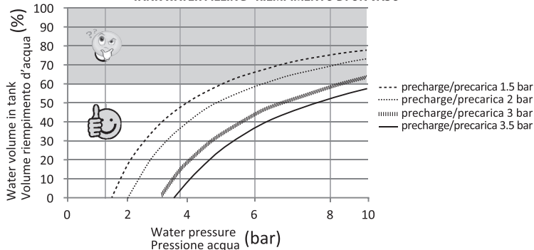
TANK WATER FILLING - RIEMPIIMENTO DI UN VASO
