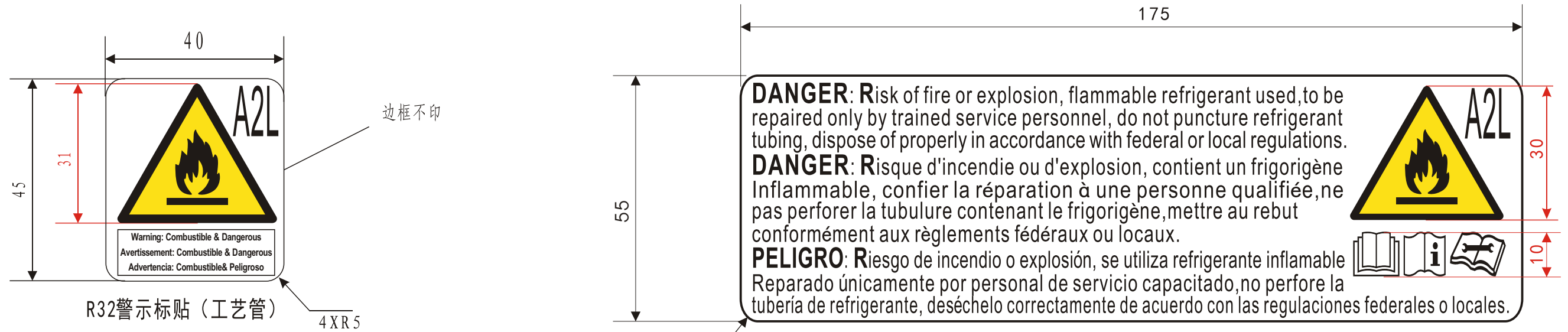
R32机身警示标贴 81102-030632改图
