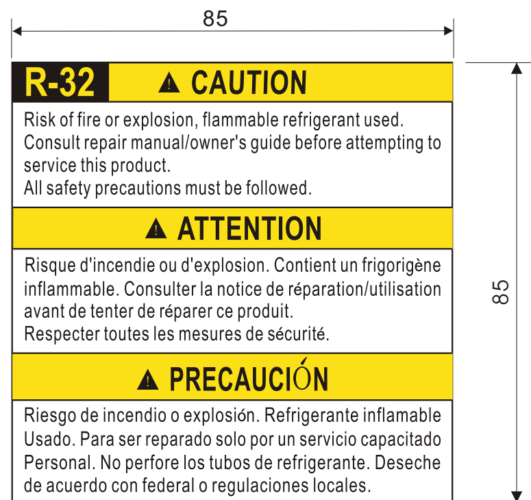
警告标识 (压机缸体)
