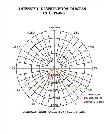
AVS-AI1-120W
