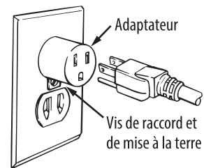
Coffret de prise de courant à contact de mise à la terre
