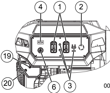
Figura 2-3. Panel de control de PM9400E con arranque eléctrico
