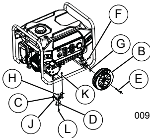
Figura 2-10. Conjunto de pata y rueda
