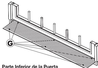
Parte Inferior de la Puerta con Barra Inferior y Placa del Umbral Instaladas
