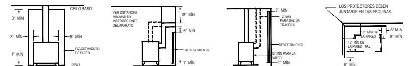
PARED SENCILLA PROTEGIDA
