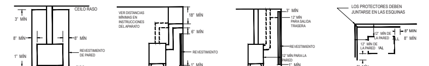
PARED SENCILLA PROTEGIDA
