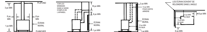
PROTECTION D'UN SEUL MUR
