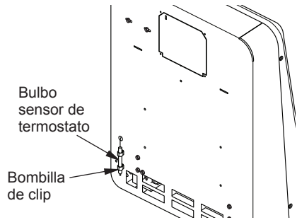
Figura 5 - Mover bulbo sensor de termostato
