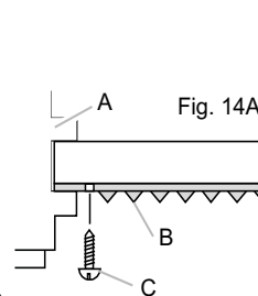
Fig. 14A A. Canal de ventana B. Cortina izquierda C. Tornillos cabeza redonda de 10 x 3/4" (o 1/2")
