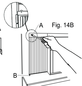
A. Tornillos cabeza redonda de 10 x 3/4" (o 1/2") B. Orificio ranurado en la parte inferior de la cortina
