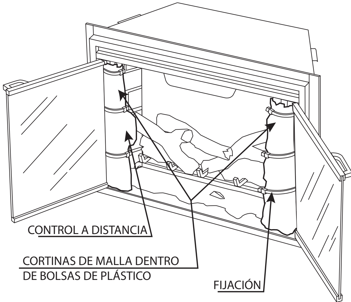
Diagrama de instalación previa: Figura 1
