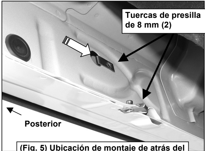
(Fig. 5) Ubicación de montaje de atrás del lado del conductor
