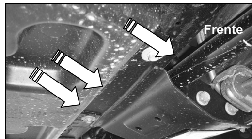
(Fig. 9) Frente del lado del pasajero ilustrado con la cubierta del tanque DEF. Retire (3) los pernos hexagonales para extraer la cubierta
