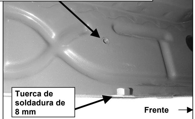
(Fig. 2) Soporte de montaje del tubo del lado del pasajero
