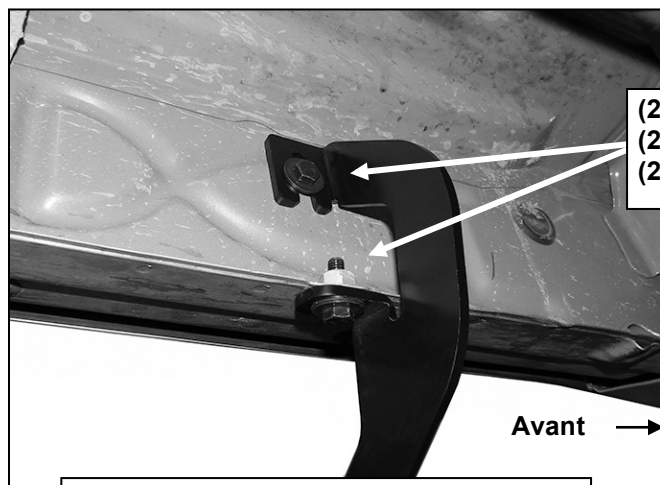
(Fig. 6) Installation du support avant gauche/côté conducteur
