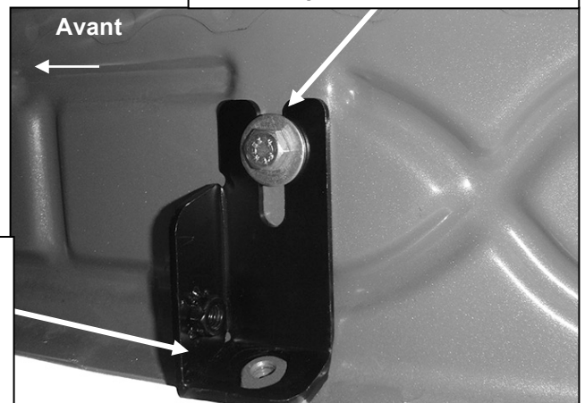
(Fig. 12) Faire glisser le support supérieur sur l'écrou soudé (s'il en est équipé - voir la figure 2)
