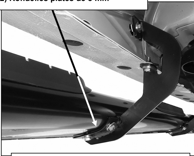
(Fig. 17) Illustration de l'installation côté passager
