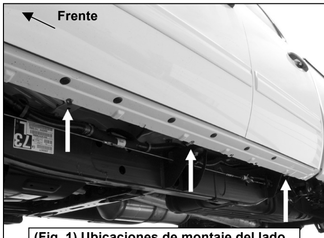
(Fig. 1) Ubicación de montaje del lado del conductor (3)
