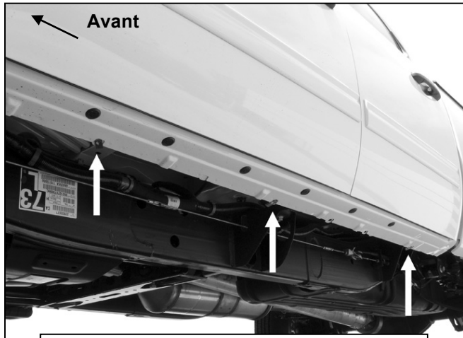
(Fig. 1) (3) emplacements de montage côté conducteur
