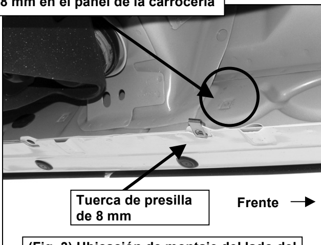
(Fig. 3) Ubicación de montaje del lado del conductor (2)
