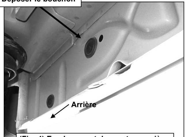
(Fig. 4) Emplacement de montage arrière côté conducteur
