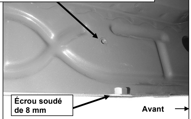
(Fig. 2) Emplacement du montage avant côté passager
