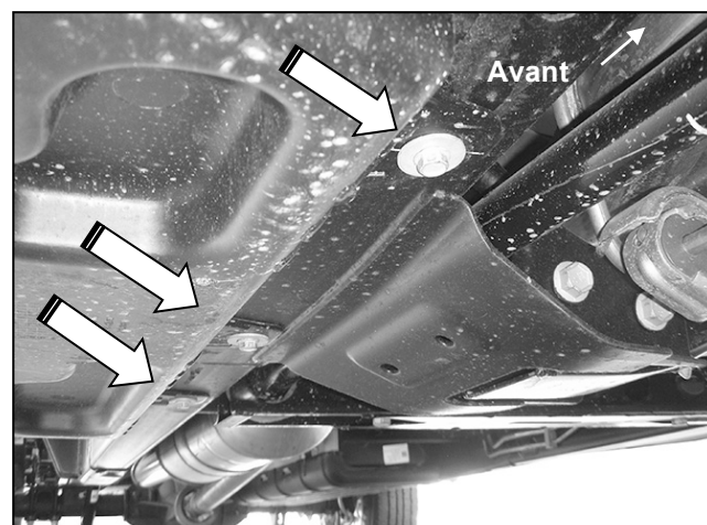
(Fig. 9) Illustration de l'avant côté passager avec couvercle du réservoir FED. Démontez les (3) boulons 6 pans pour retirer le couvercle
