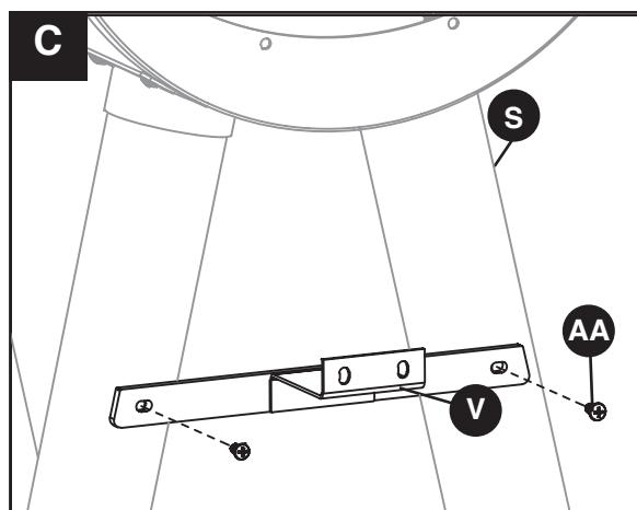
DGSS675CB-D Bracket
