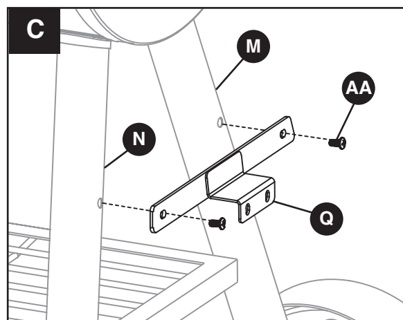
DGSS443CB-D abrazadera de soporte
