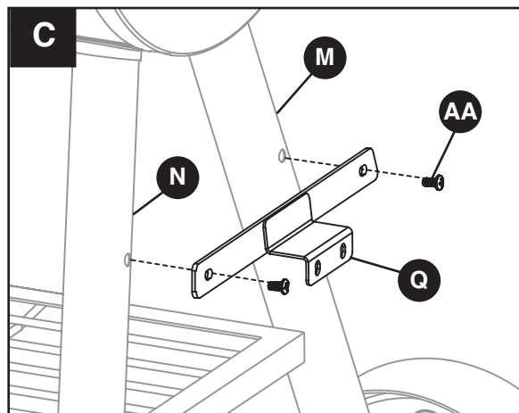
DGSS443CB-D Bracket
