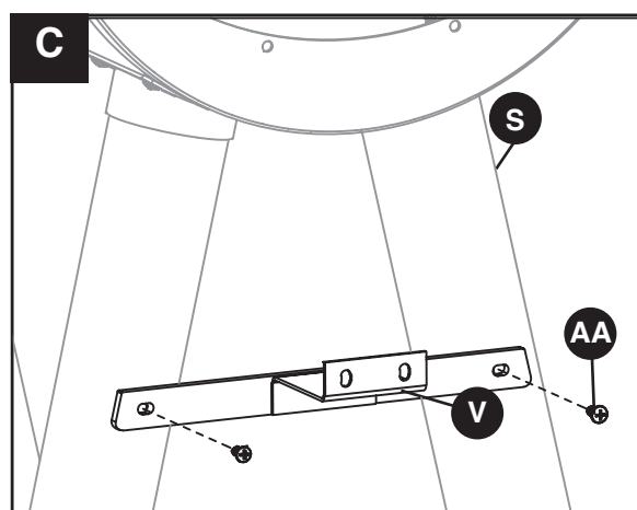
DGSS675CB-D abrazadera de soporte
