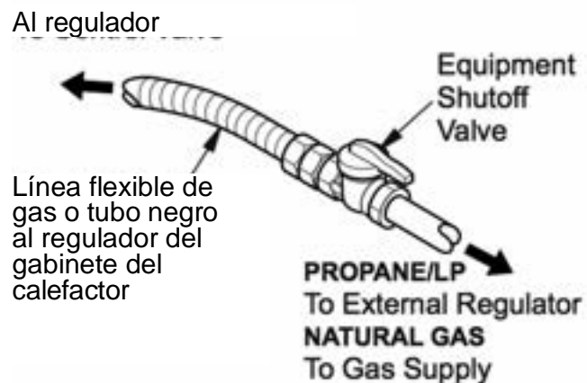
Fig. 11 - Instalación de la línea flexible de gas a la válvula de cierre del equipo
