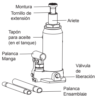
FIGURA 1: gato de botella común
