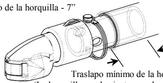
Traslapeo mínimo de la horquilla - 7"
