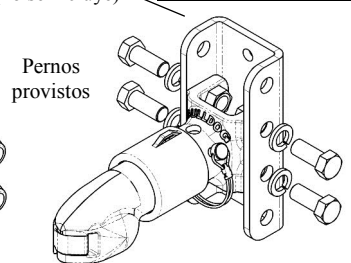
Canal de 3.0" (no se incluye)
