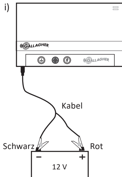
Mit dem Leitungs-Kit (G58210) an eine 12-Volt-Batterie
