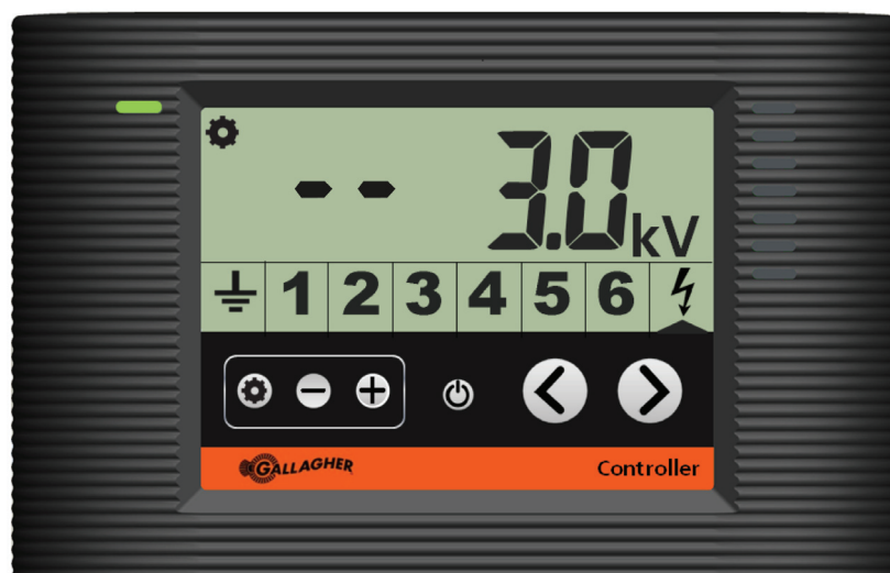
Der Display Controller zeigt die Standard Alarmeinstellung des Weidezaungerätes mit ausgeschaltetem Strom und Spannung bei 3,0 KV
