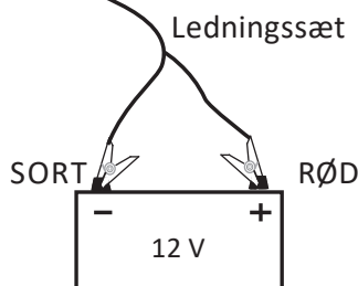
12 V batteri via ledningssæt (G58210)
